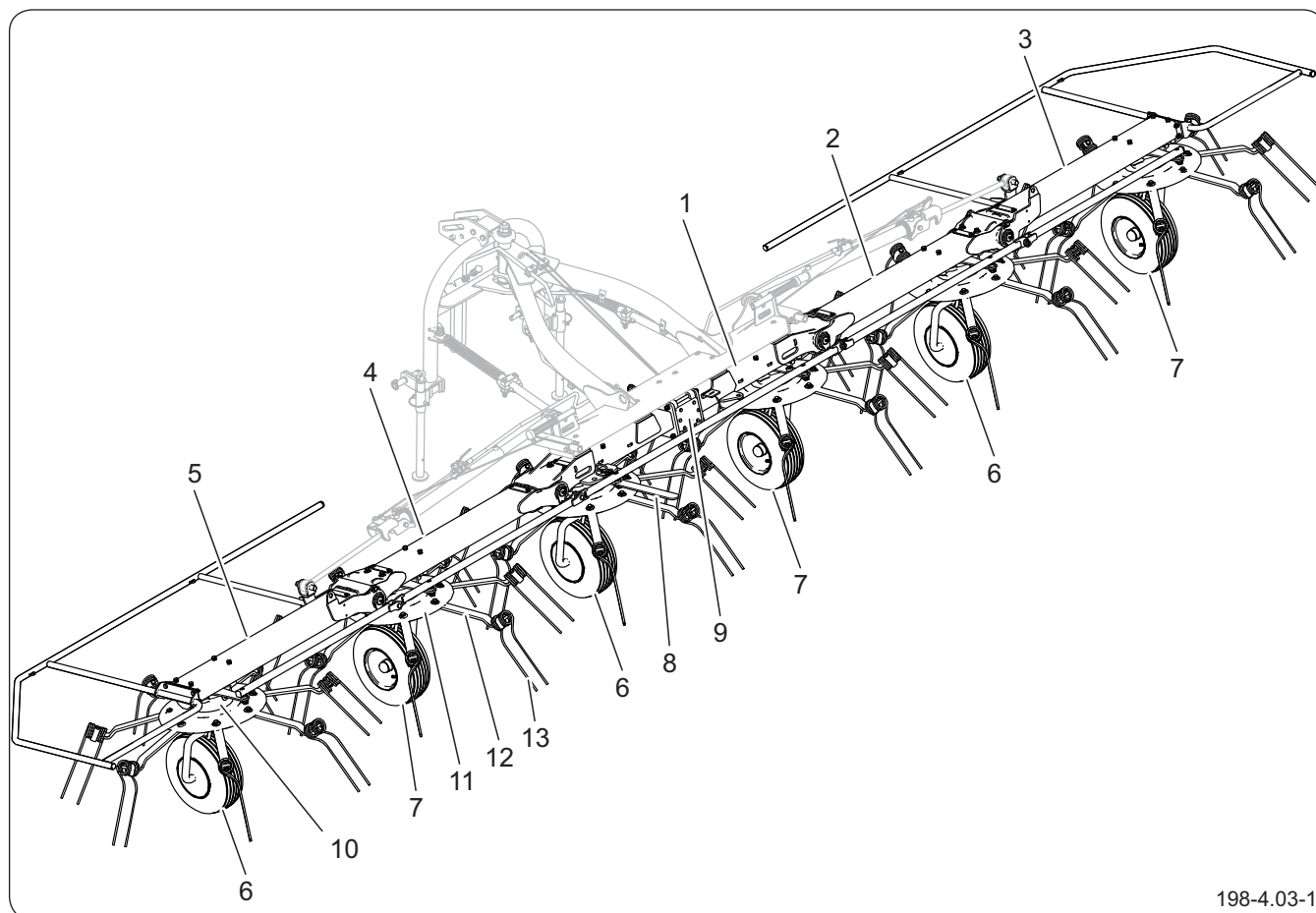
Рисунок 4.3 Конструкция модуля
