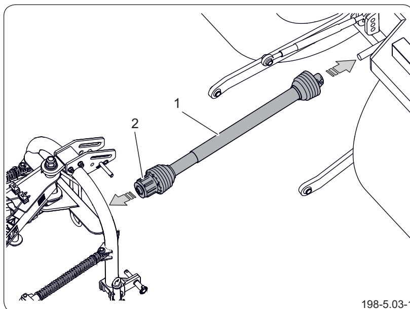
Рисунок 5.2 Телескопический карданный вал с предохранительной муфтой
