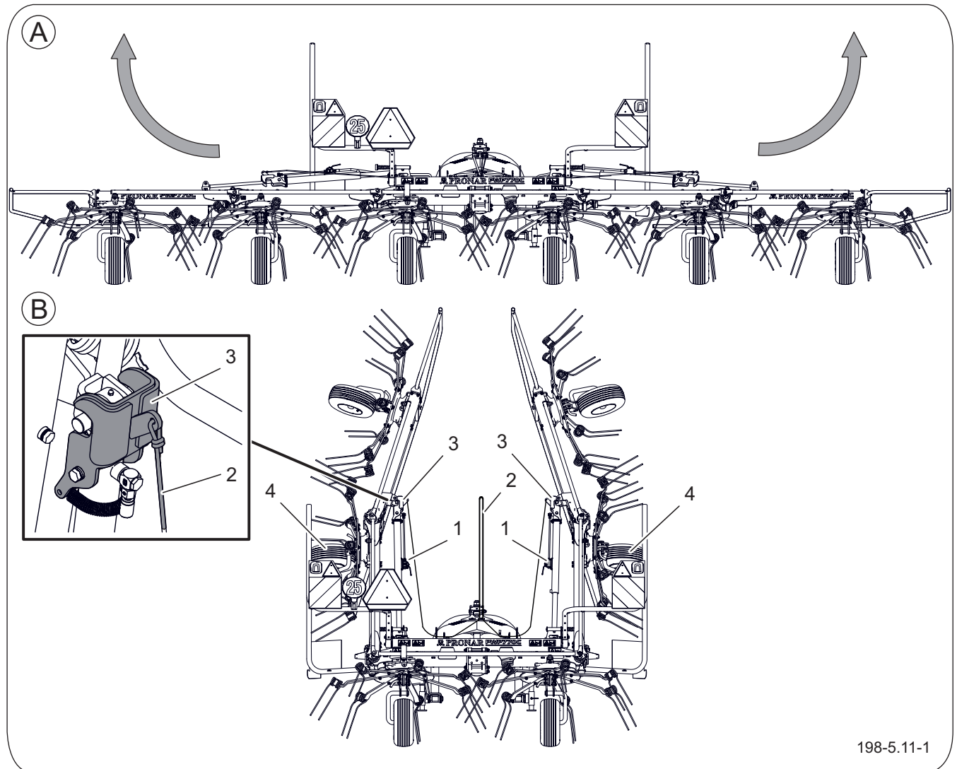
Рисунок 5.15 Положения ворошилки-вспушивателя
