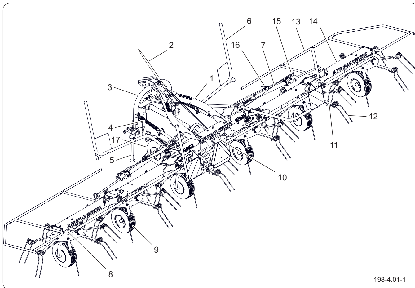
Рисунок 4.1 Устройство машины
