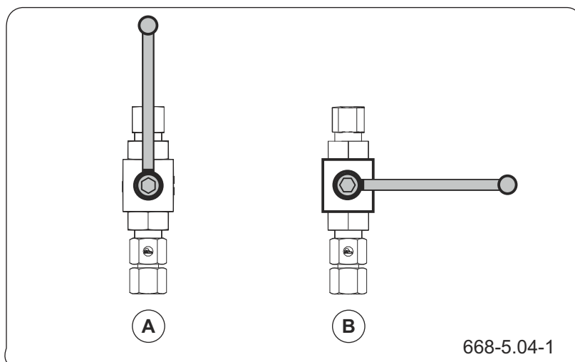
Рисунок 5.17 Шаровой клапан
