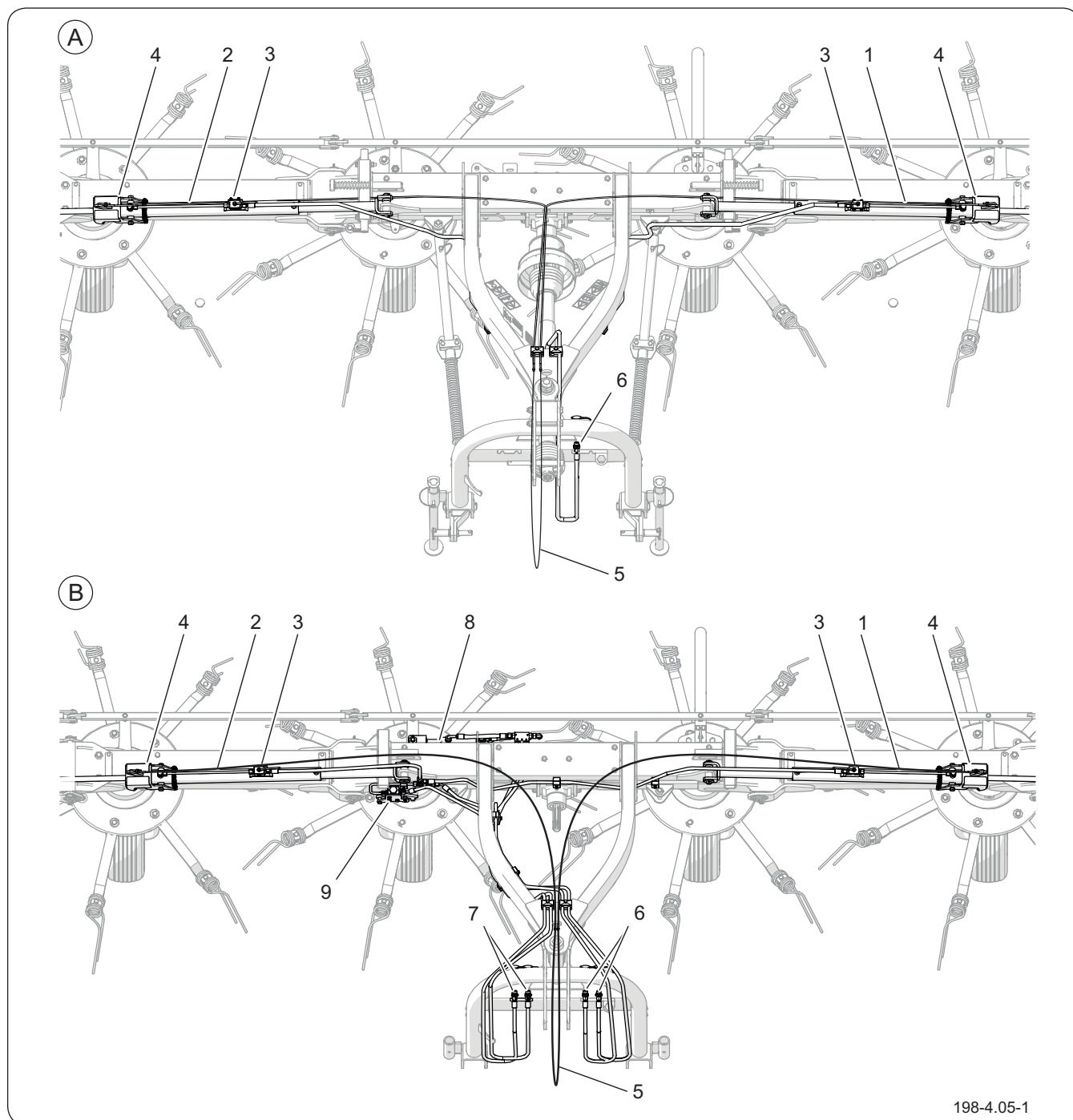
Рисунок 4.5 Устройство гидравлической системы
