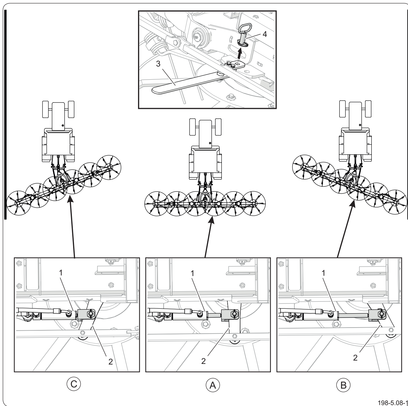
Рисунок 5.14 Граница ворошения - гидравлическое управление (дополнительное оборудование)
